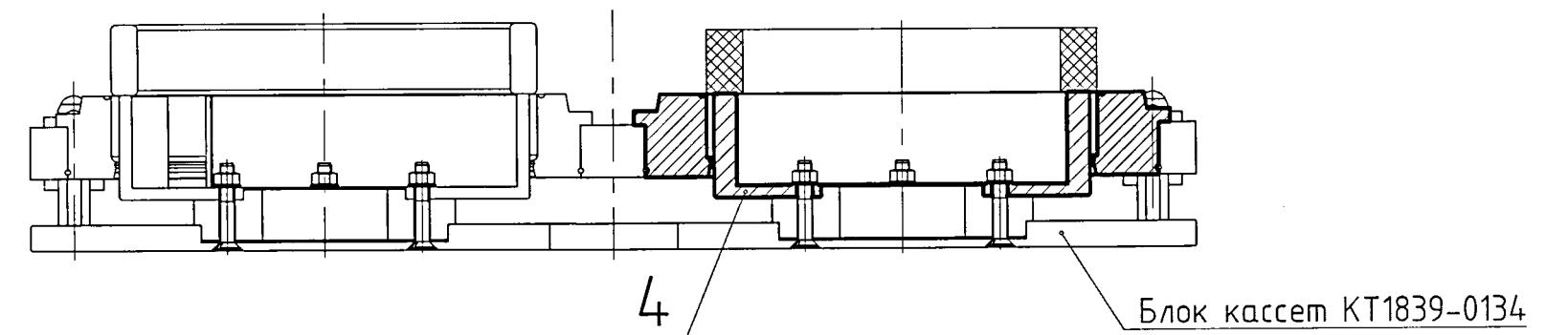
Схема извлечения изделия (1:4)
