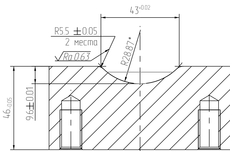
B-B
