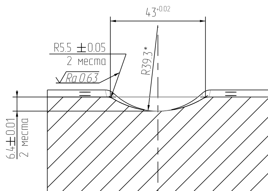
Г-Г
