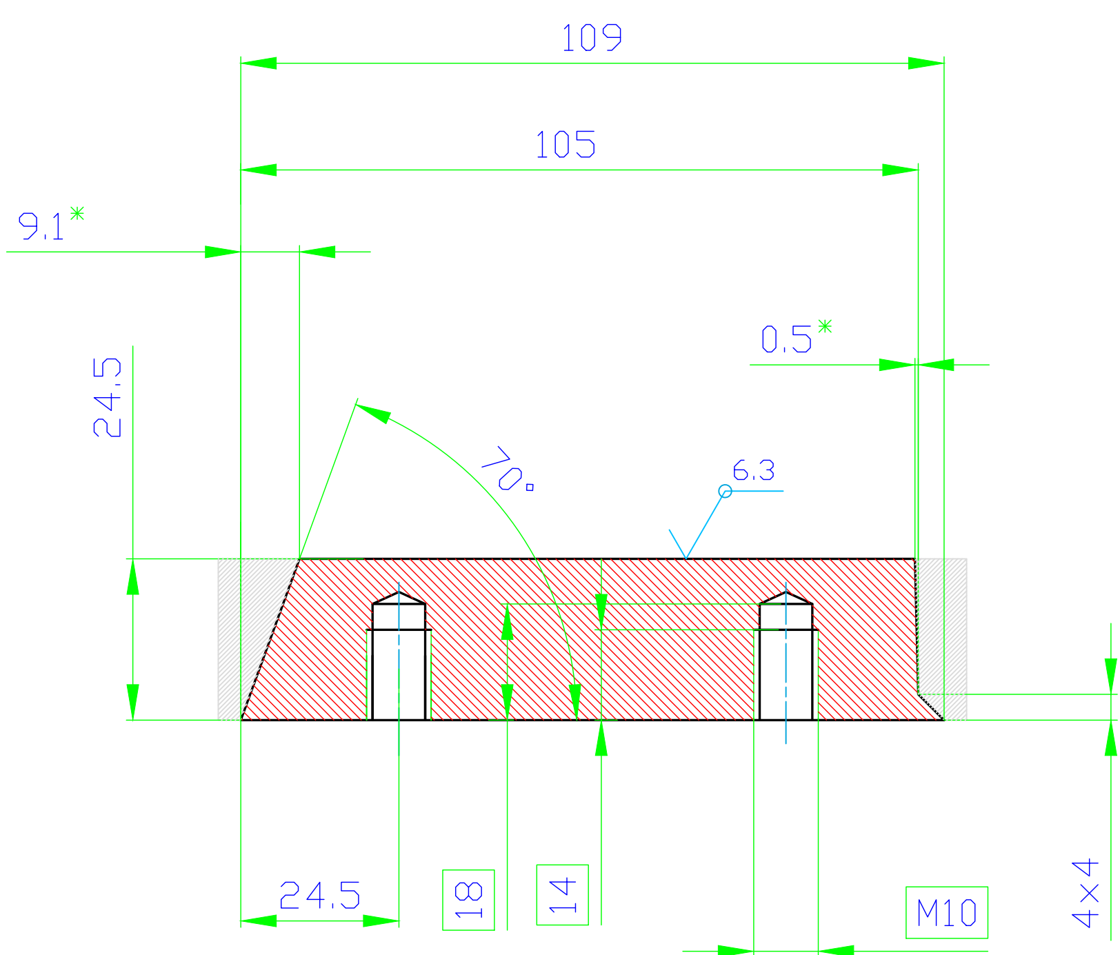
В-В(2:1)
