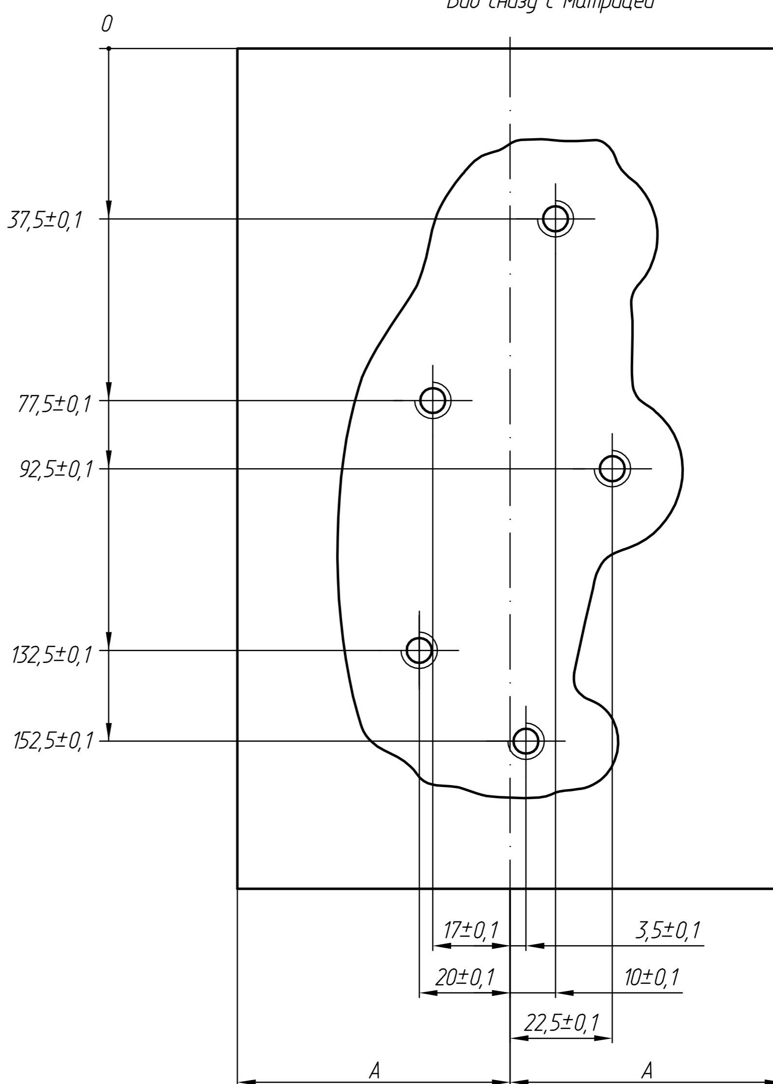
Вид снизу с матрицей
