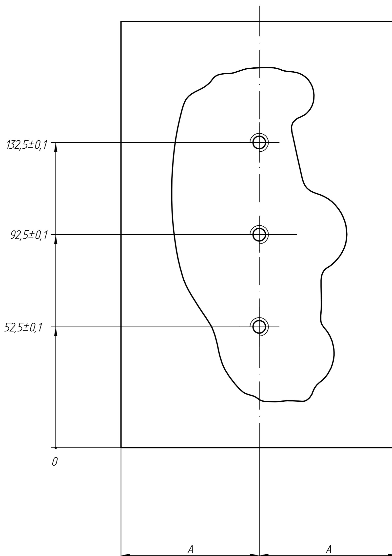
Вид сверху с матрицей
