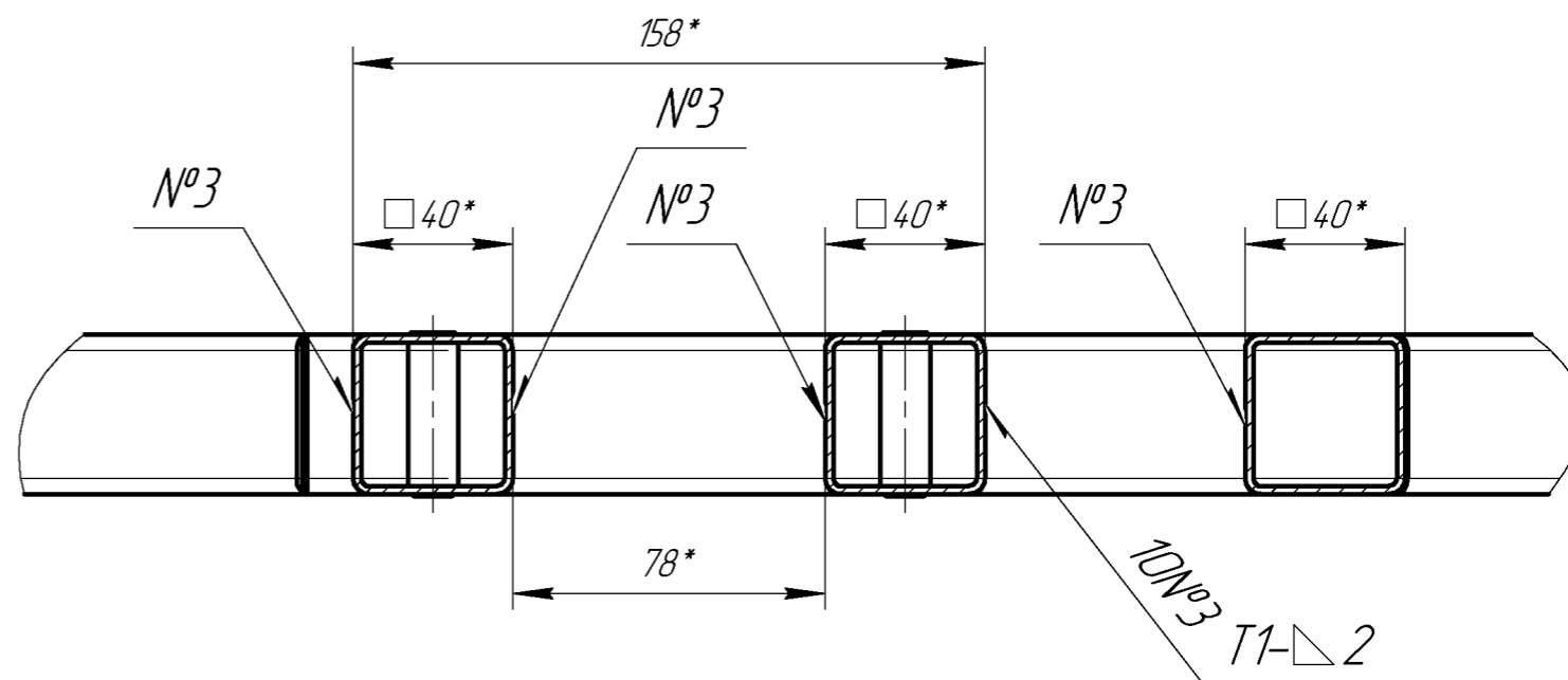
B-B(1:2)(1)
