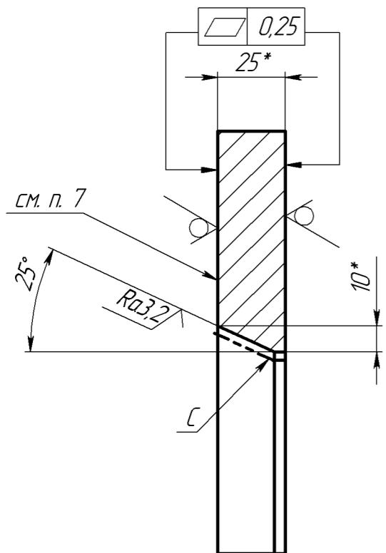
A-A (1 : 2)
