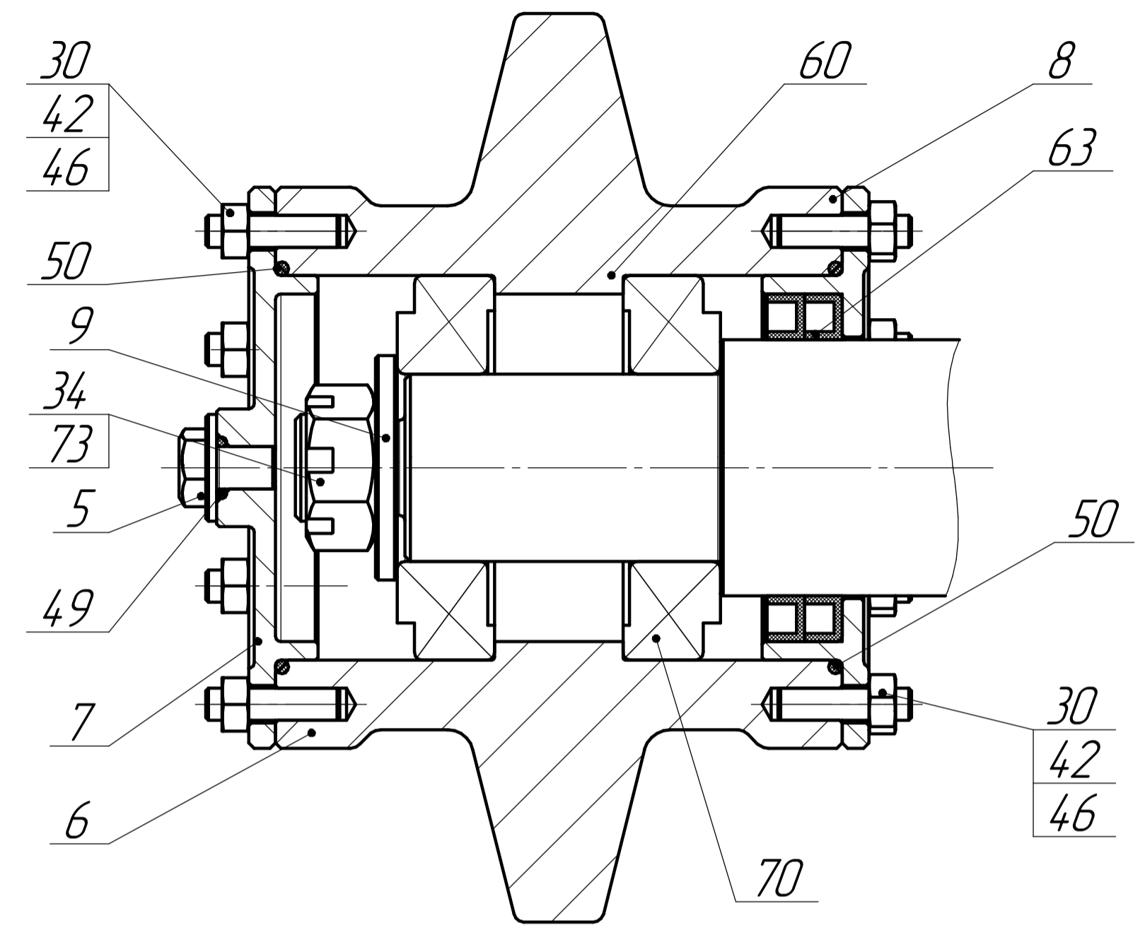
Г-Г (1:1) Ø
