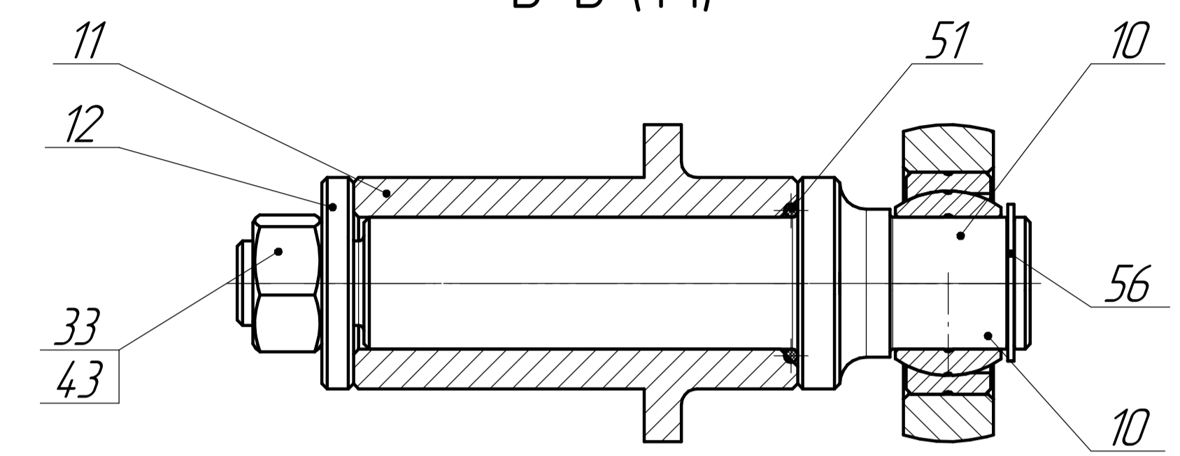
Б-Б (1:1)
