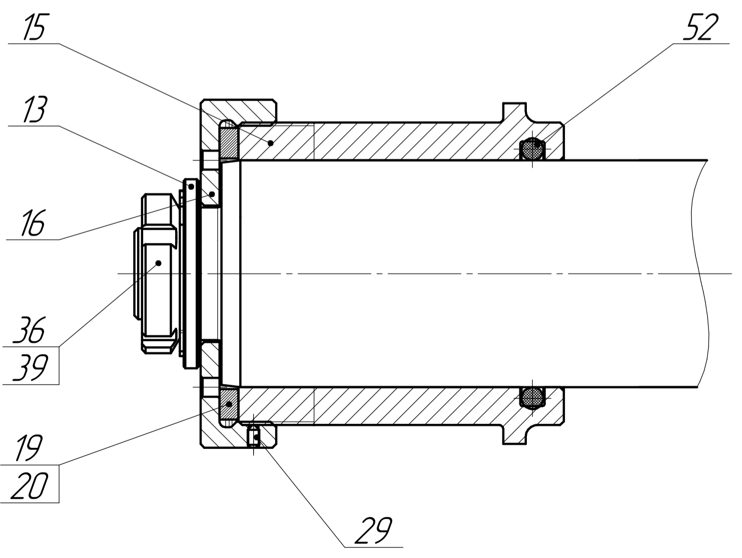
Г-Г (1:1) Ø
