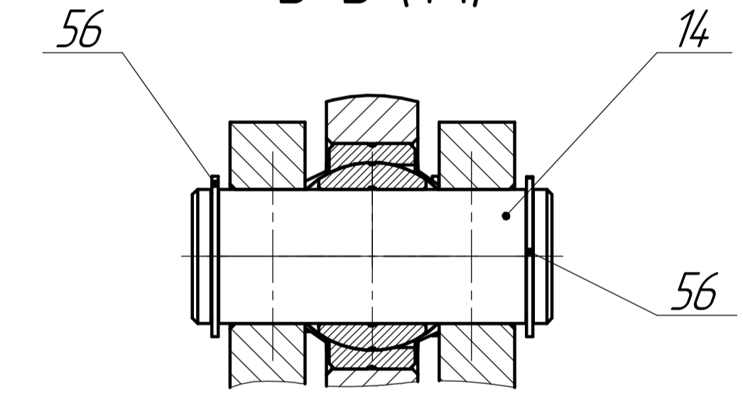
В-В (1:1)
