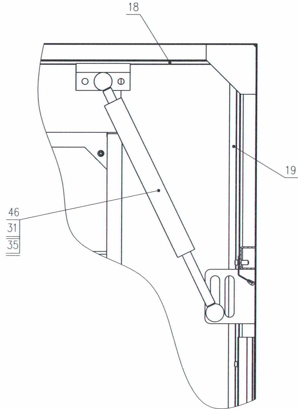
Г-Г (1:2,5)
