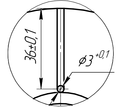
Г(1:1)
