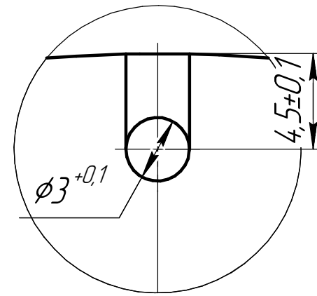
Б(4:1)
