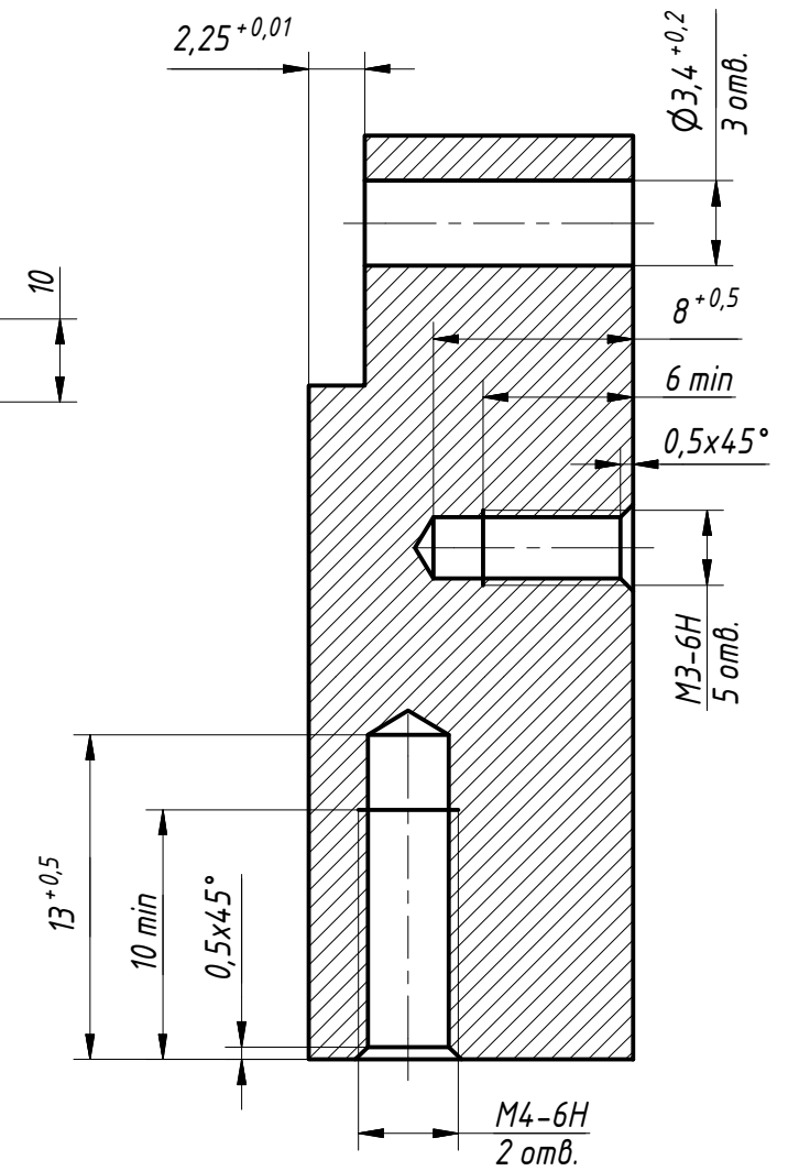
Б-Б (3:1)
