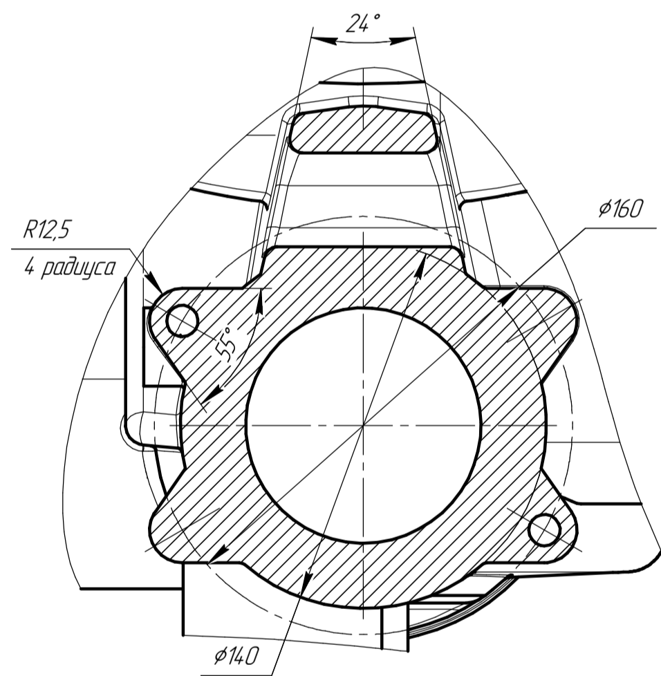
М 1 -М 1 (3)
