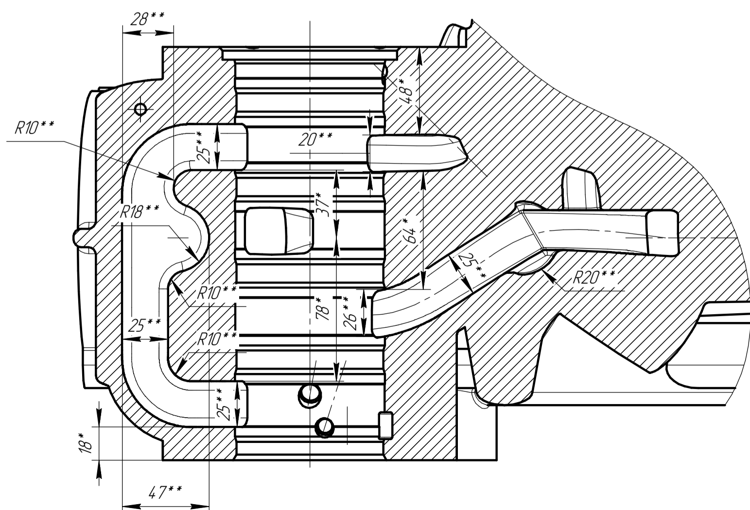
Ш 1 -Ш 1 ○(1)
