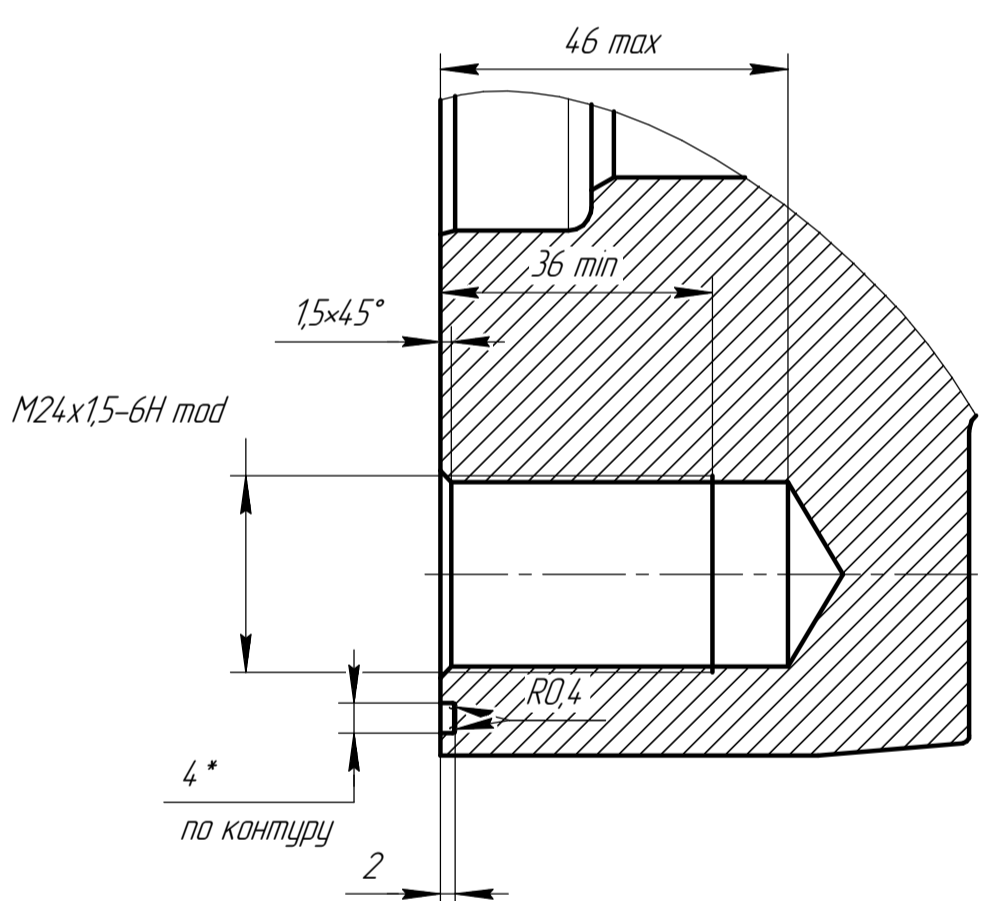
И 1 -И 1 (1:1)○(2)
