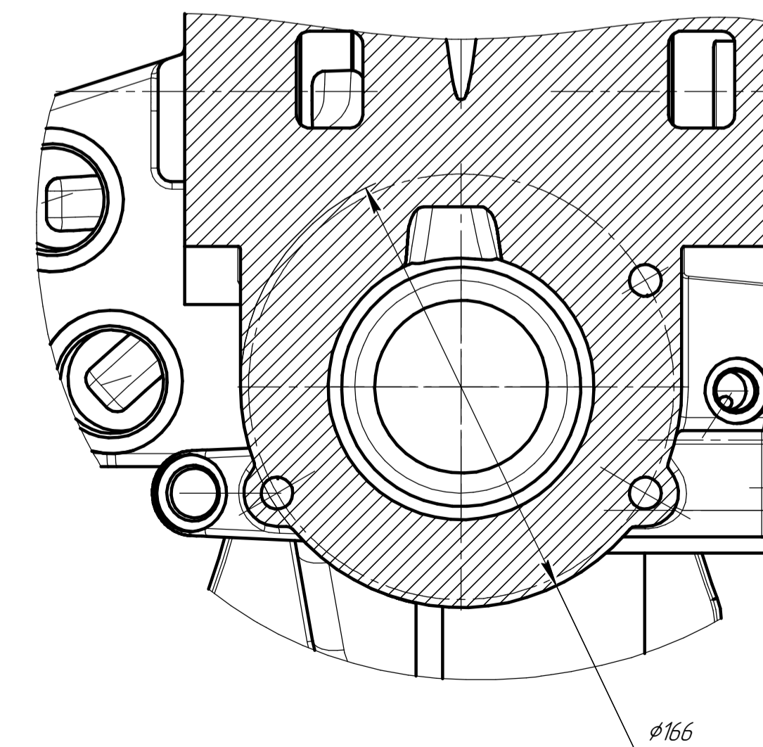
Н 1 -Н 1 (3)
