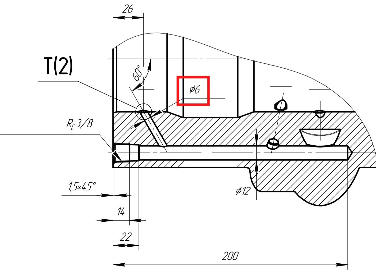
Ш-Ш○(1)
