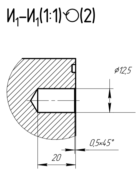
И 1 -И 1 (1:1)○(2)
