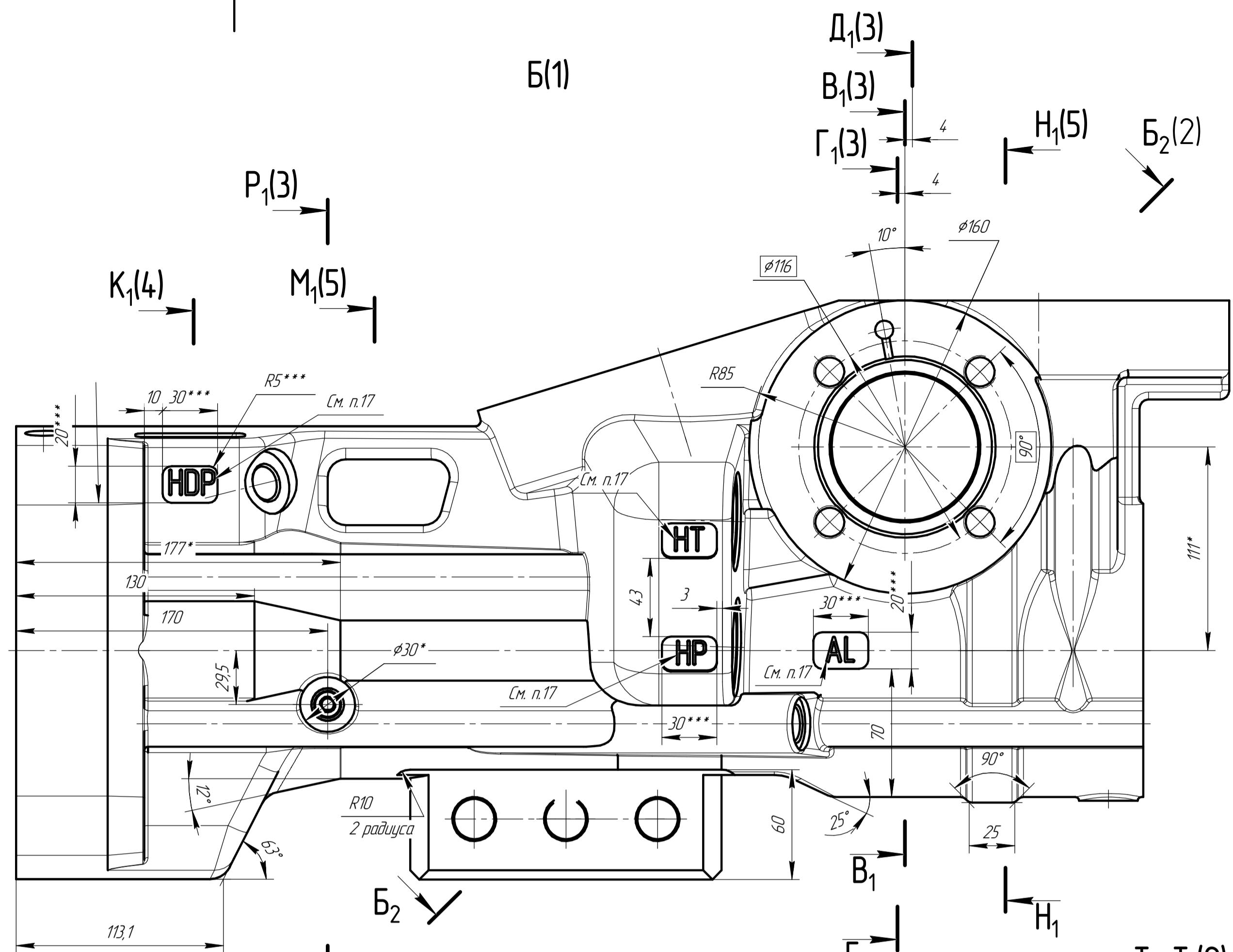
T 1 -T 1 (2)
