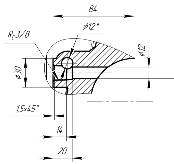
T 1 -T 1 (2)
