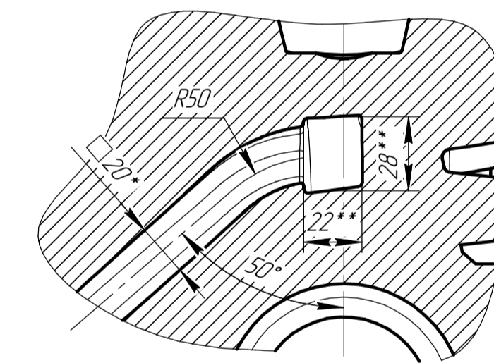
Е 2 -Е 2 (1)
