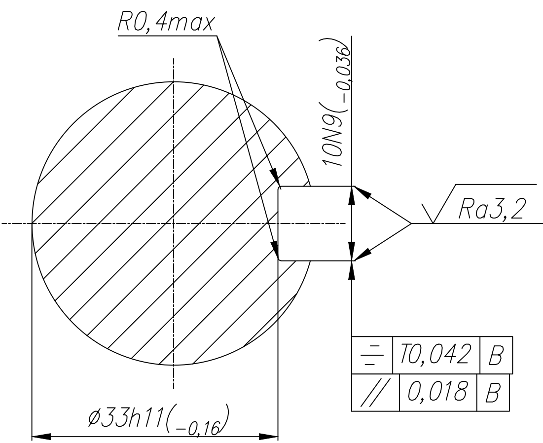
A-A (2:1)
