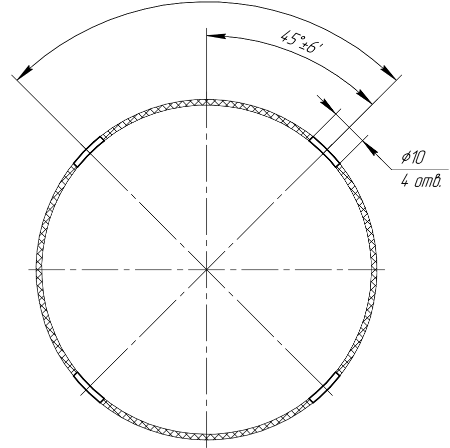
В-В 90°
