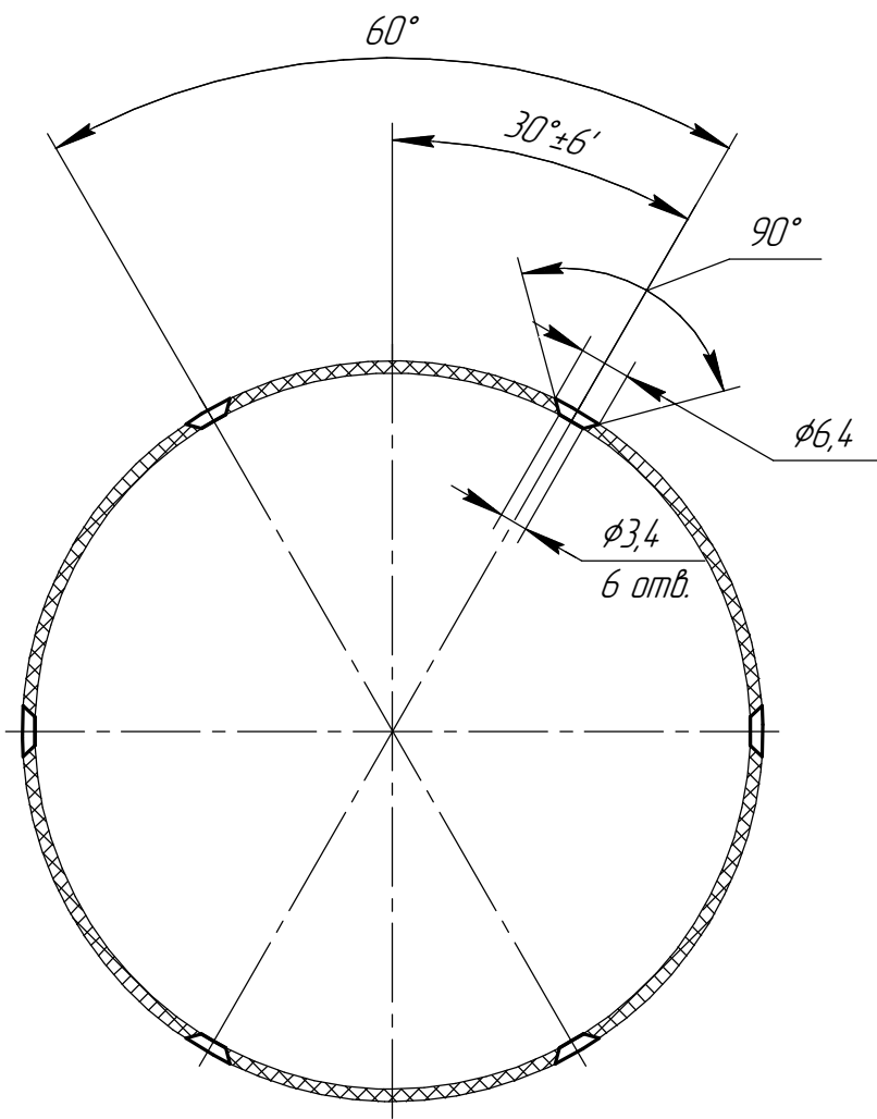
А-А 2 места
