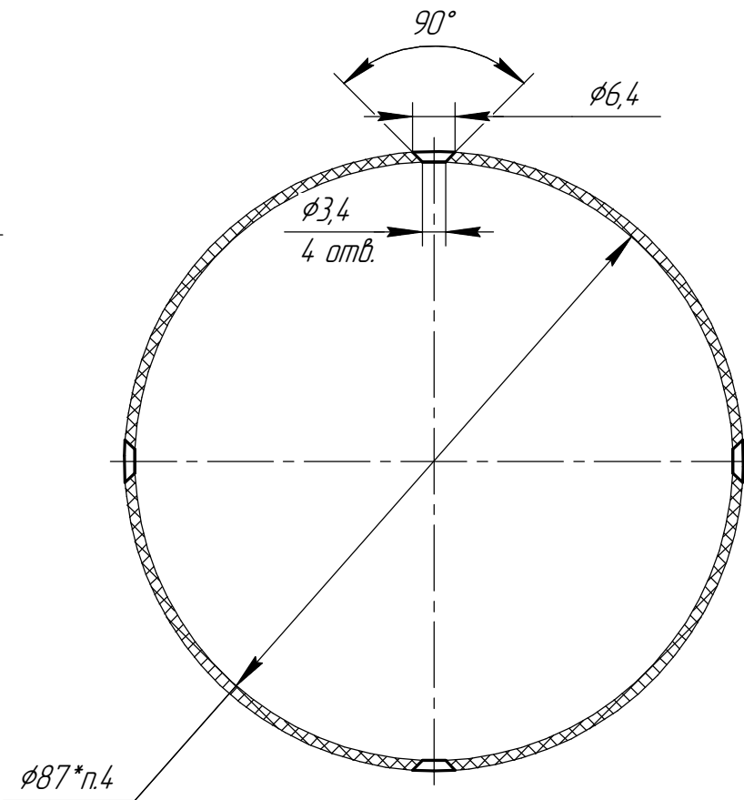
Б-Б 2 места
