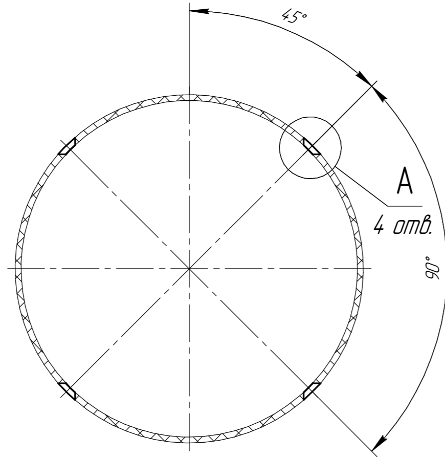
Г-Г(1:1) 2 места
