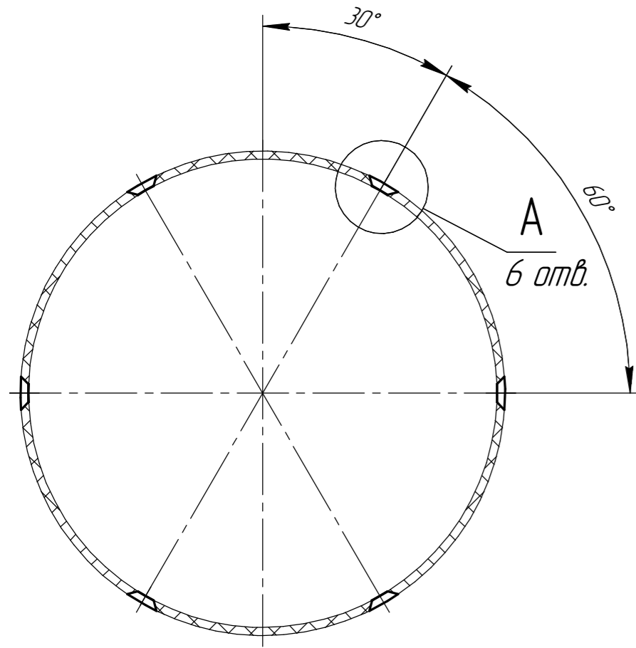
В-В(1:1) 2 места
