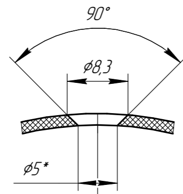
Б(2:1)⊙
