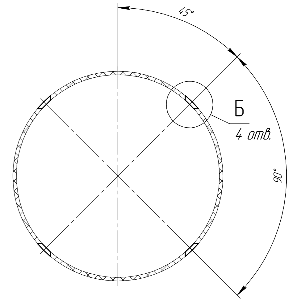
Ж-Ж(1:1)
