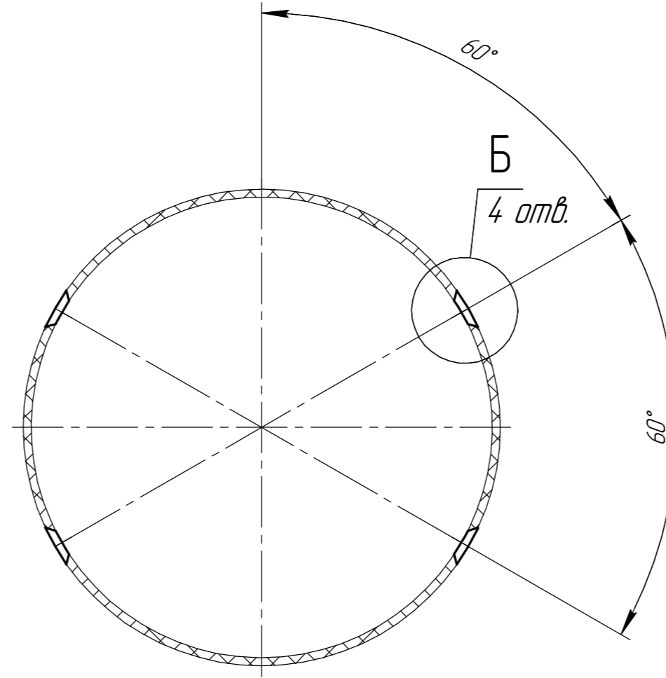
Д-Д(1:1) 2 места
