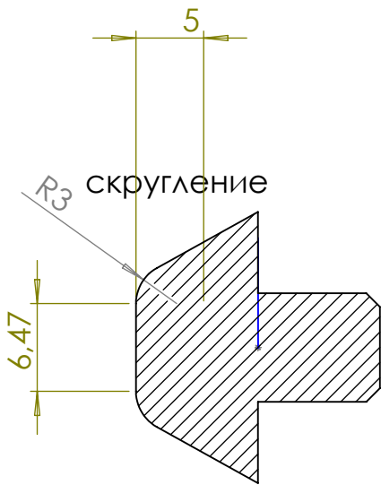
СЕЧЕНИЕ В-В
