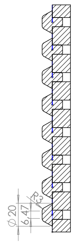
СЕЧЕНИЕ А-А
