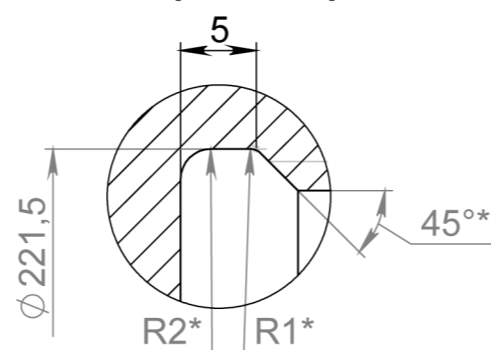
Е (2 : 1)
