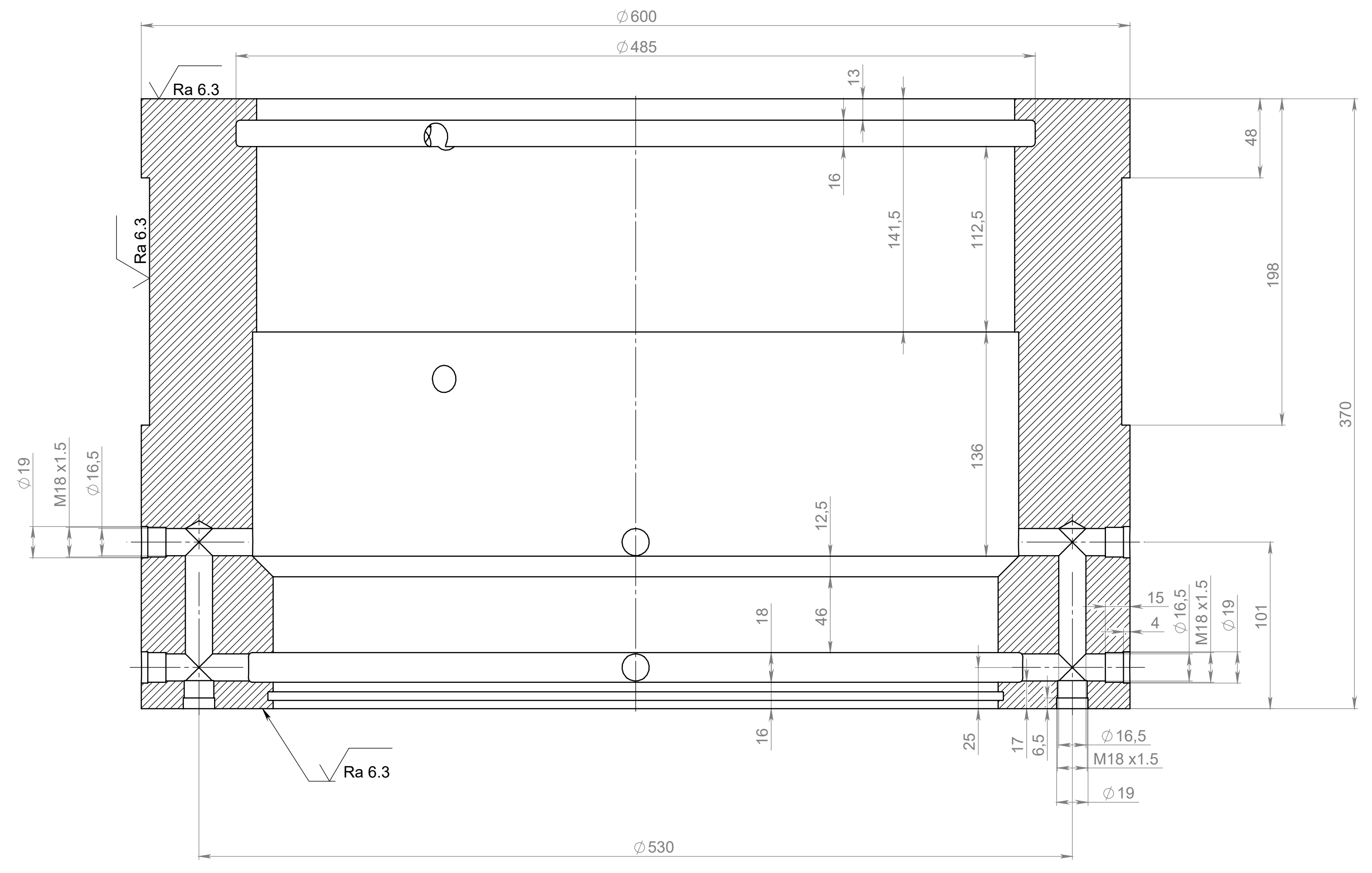
A-A (1 : 2)
