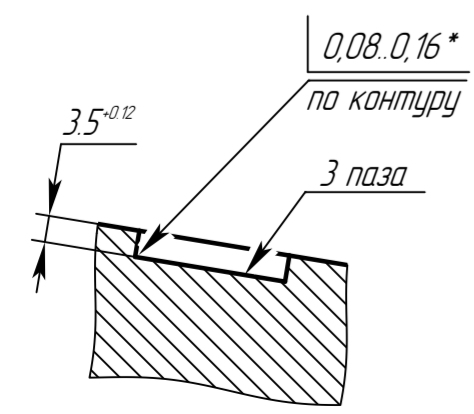
Б-Б
