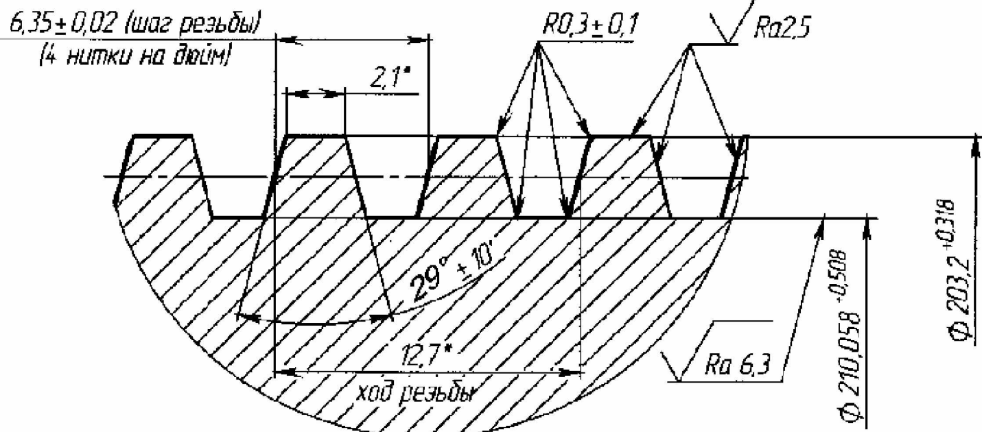
A (4 : 1) Профиль резьбы 8,25-0,25P-0,5L-ACME-2G
