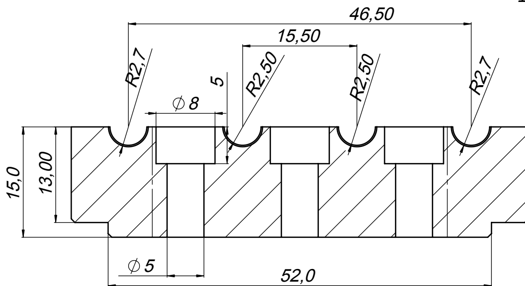
A-A (2 : 1)
