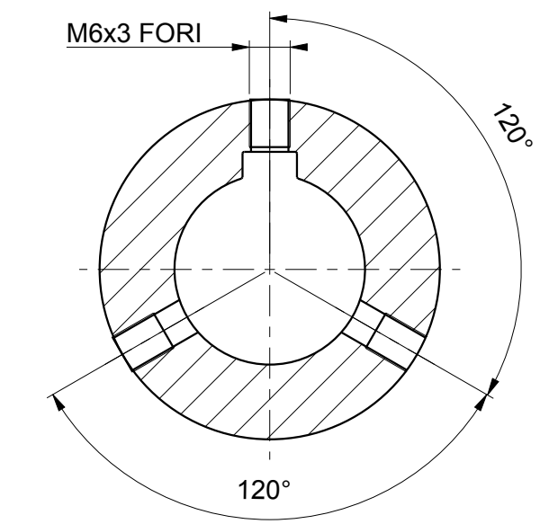
SEZIONE D-D
