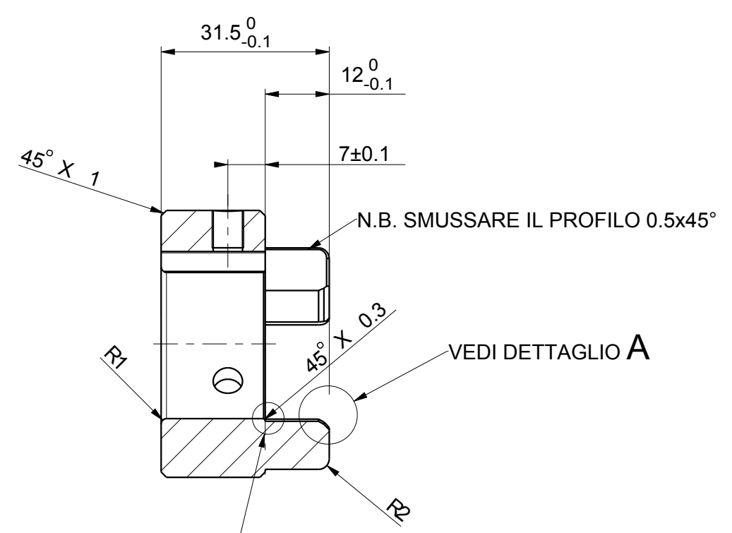
SEZIONE A-A
