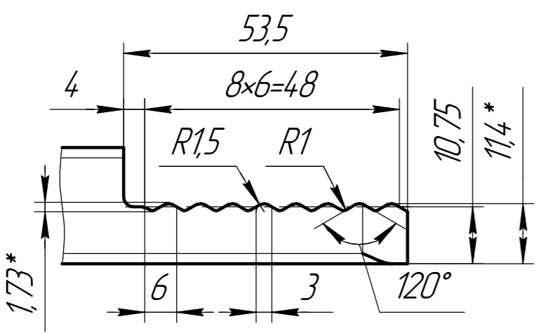
A(1:1) 2 места
