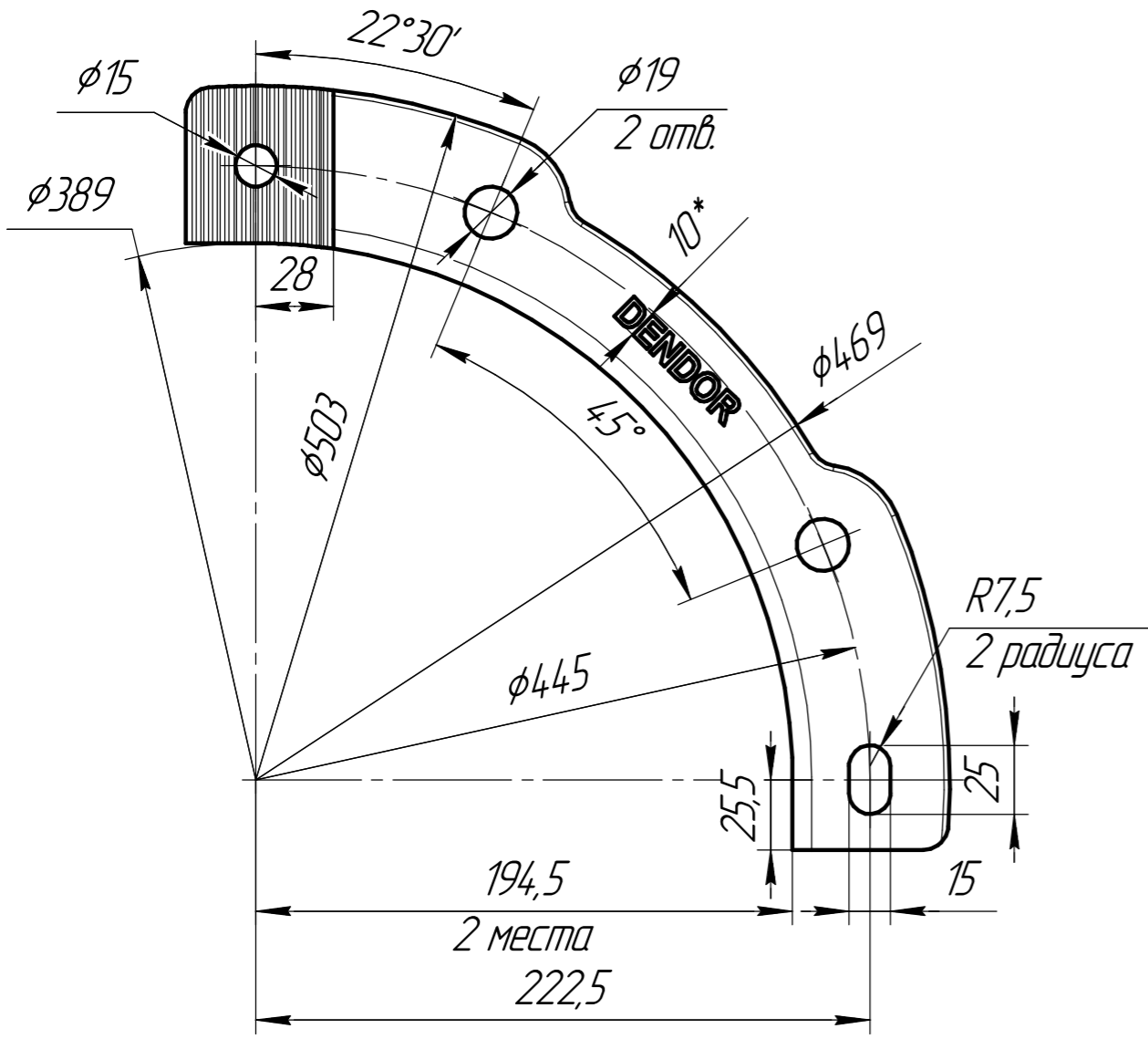
Б-Б(1:1) ☉
