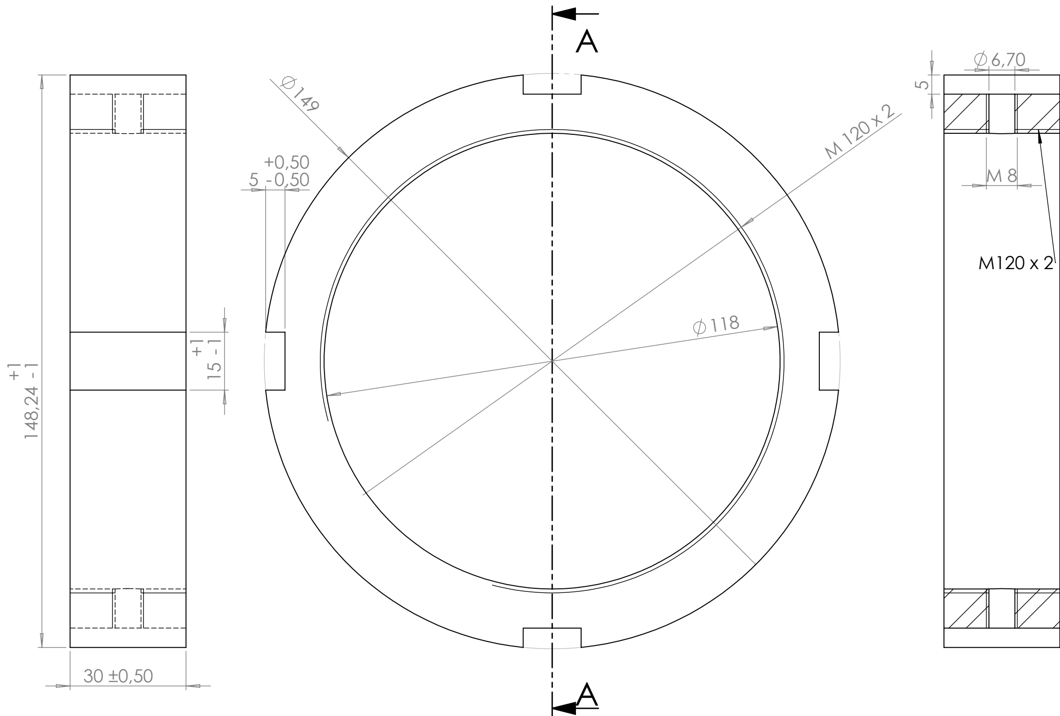
СЕЧЕНИЕ А-А МАСШТАБ 1 : 1
