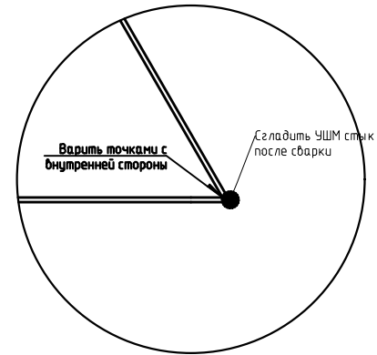
Узел А (5:1)
