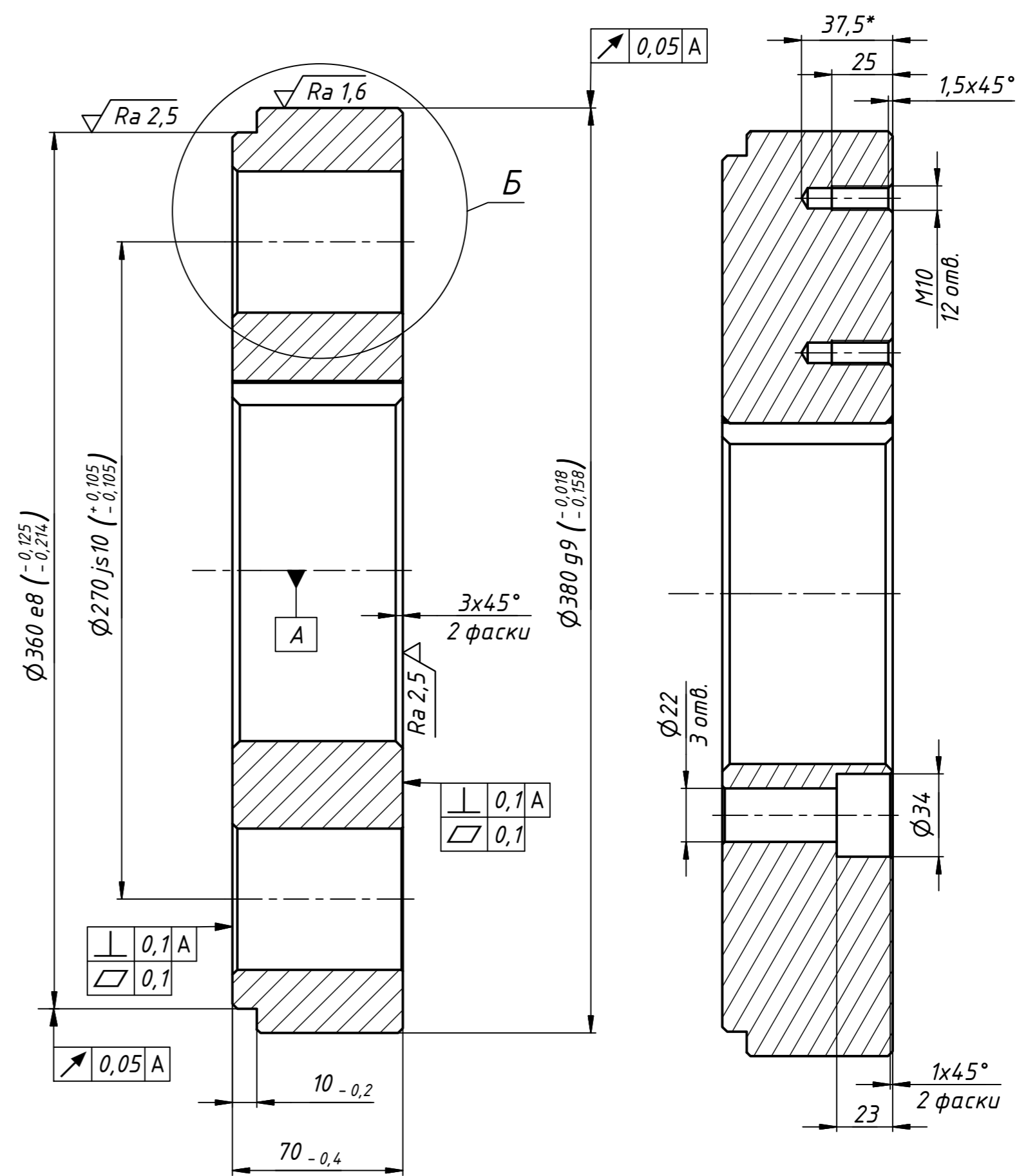
A-A (1:2)
