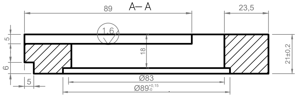
Деталь 3Б.- 1 шт сталь 45
