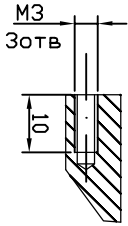
А-А
