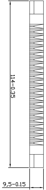
Вид Б
