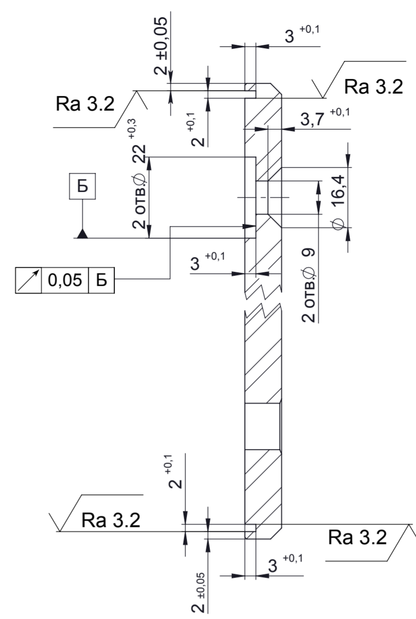
Ж-Ж, 3-3 (1 : 1)
