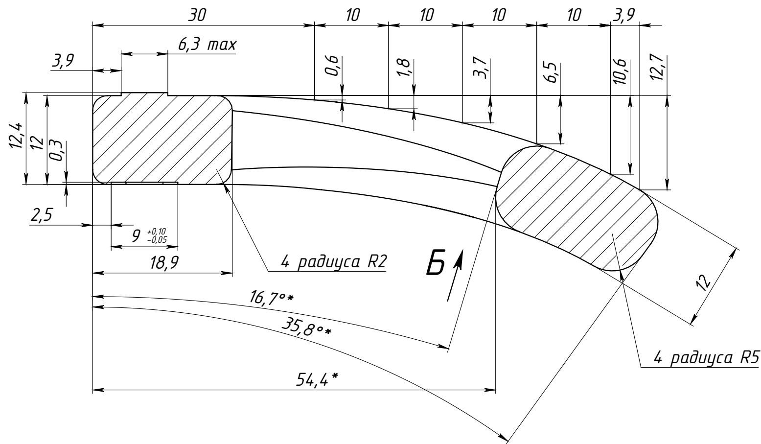
А-А (2 : 1)
