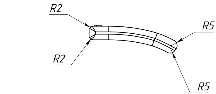
А-А (2 : 1)
