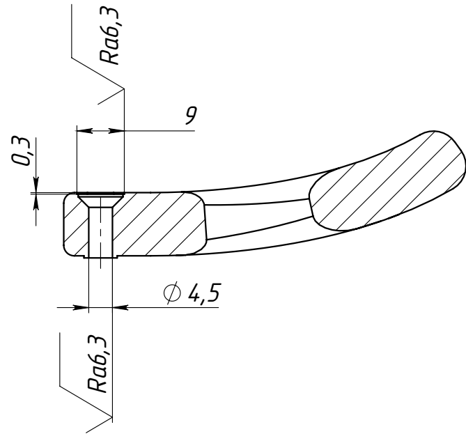
Г-Г (1 : 1)
