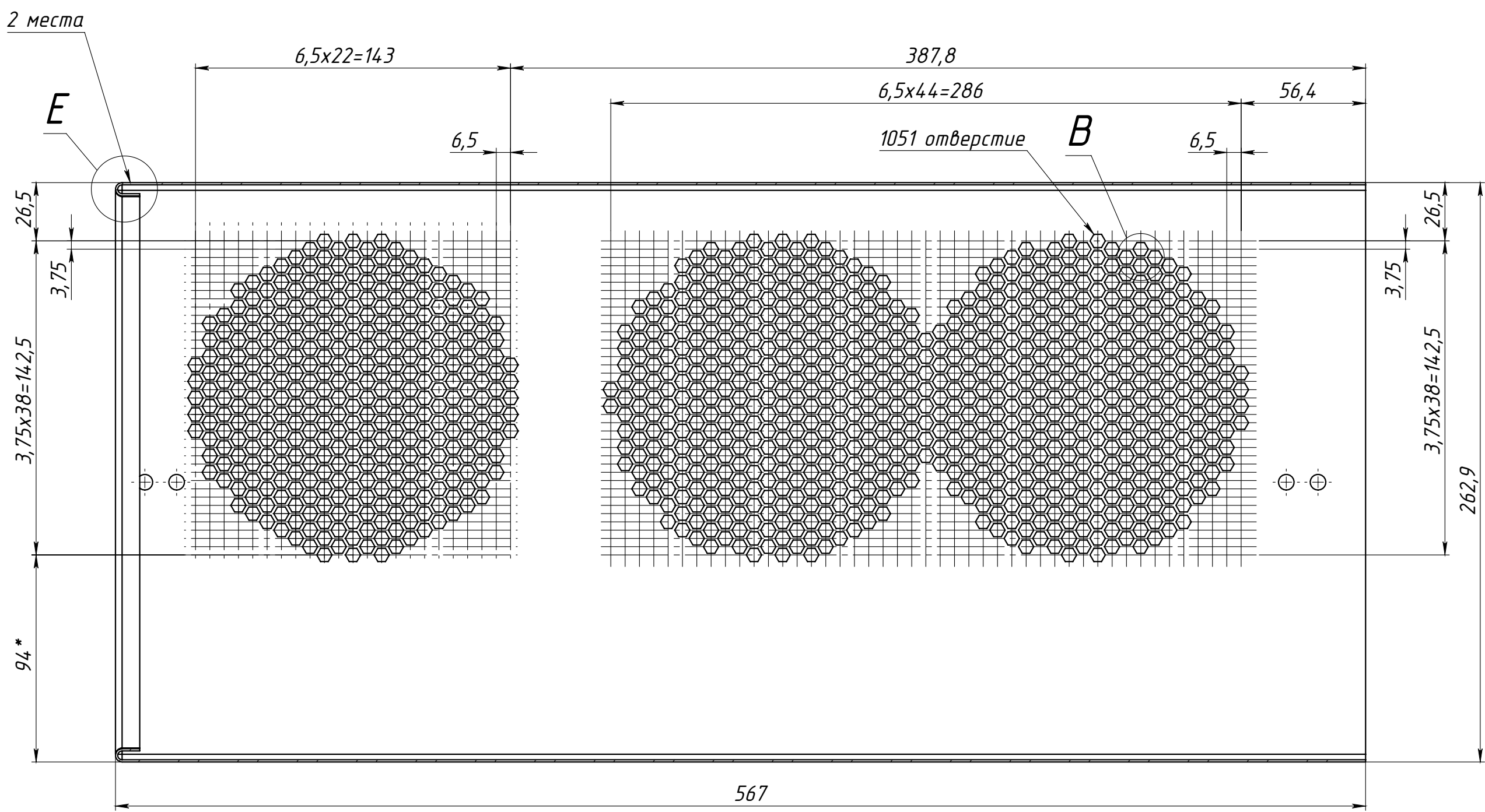
Б-Б (1 : 2)
