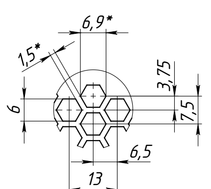
В (1 : 1)
