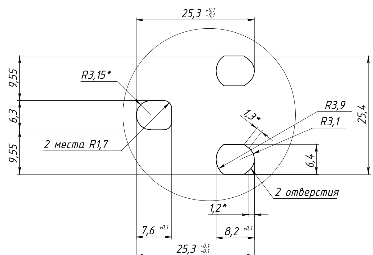
З (2 : 1)
