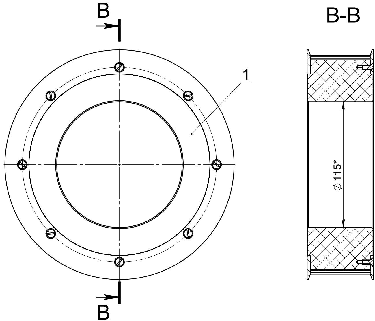
Изображено - 015.00.02.010-01 - Шкив АТ20 Z=32 В=50
