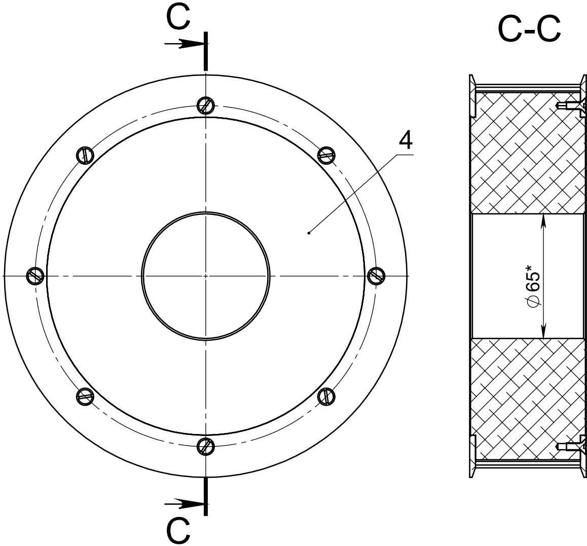
Изображено - 015.00.02.010-02 - Шкив АТ20 Z=32 В=50
