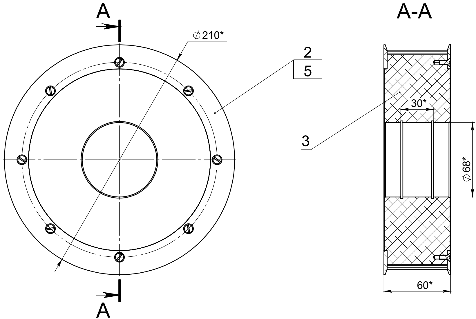
015.00.02.010 - Шкив АТ20 Z=32 В=50 - Изображено
