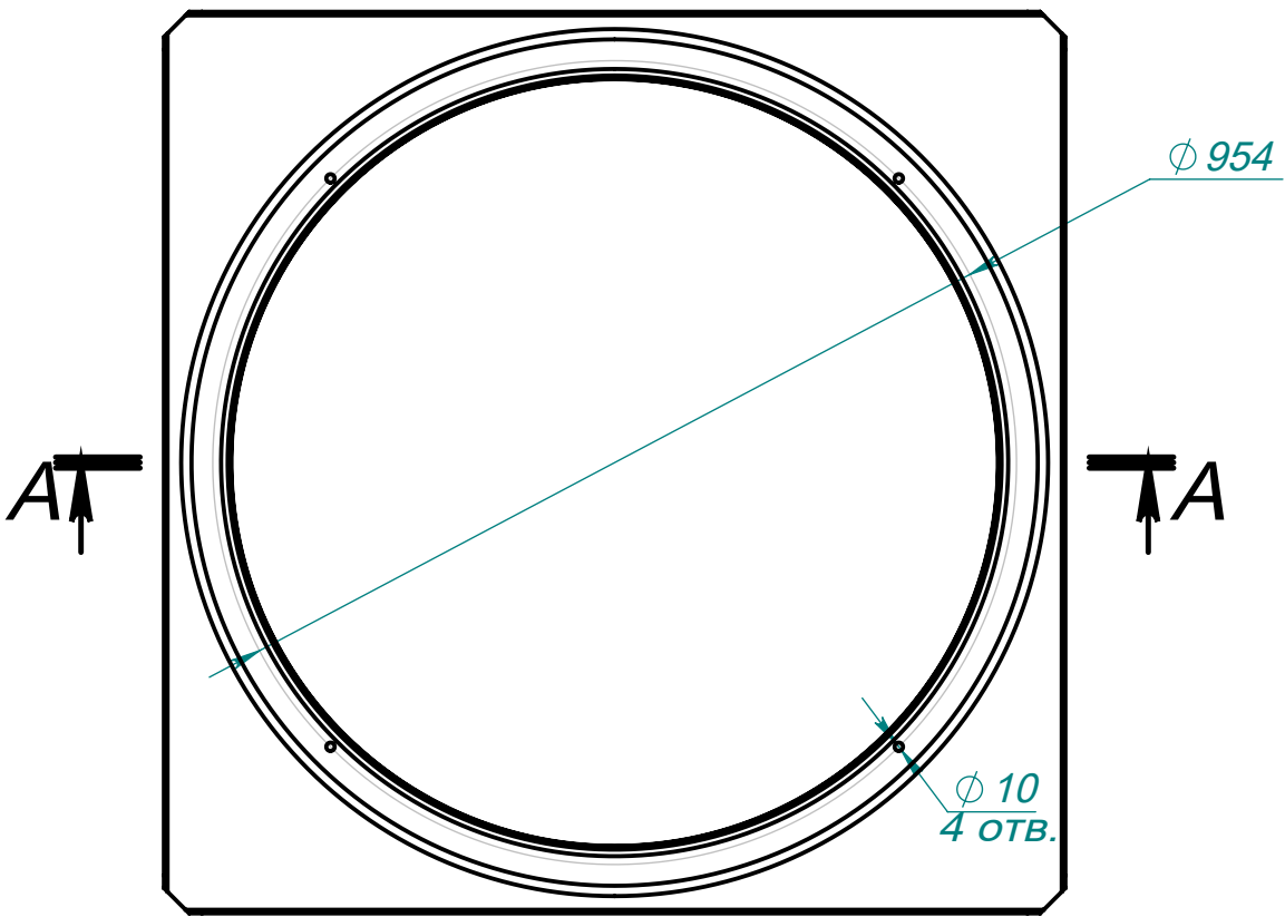
A-A (1 : 3)
