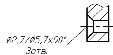
Б-Б(2:1)
