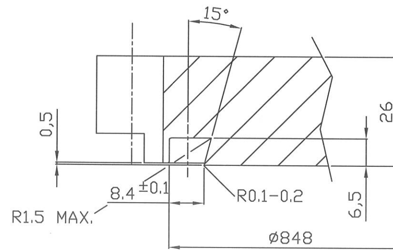
O RING GROOVE DTL
