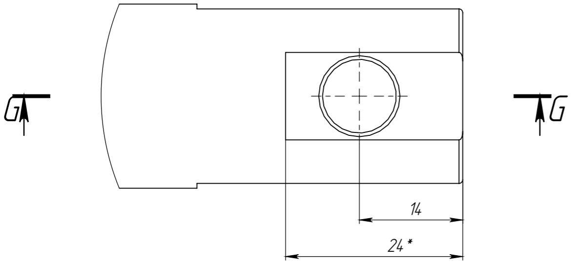
G-G (2 : 1)
