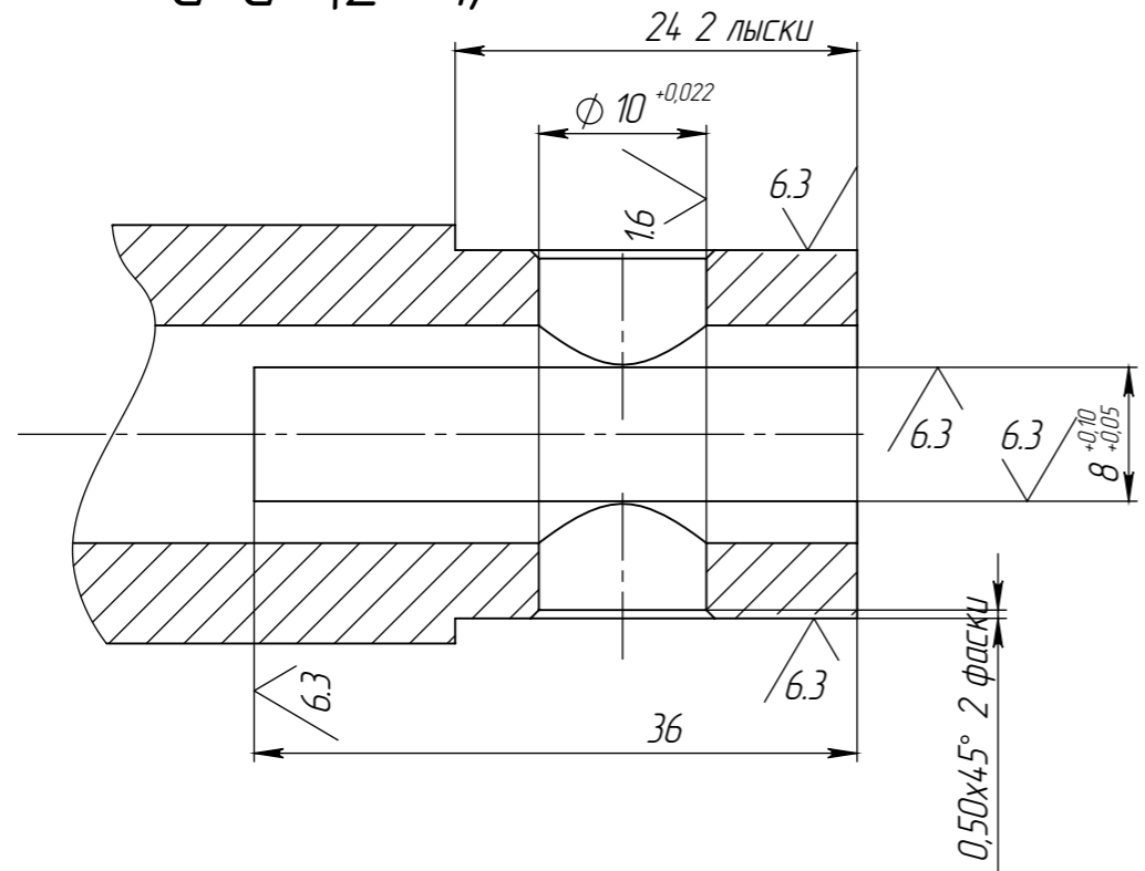
G-G (2 : 1)
