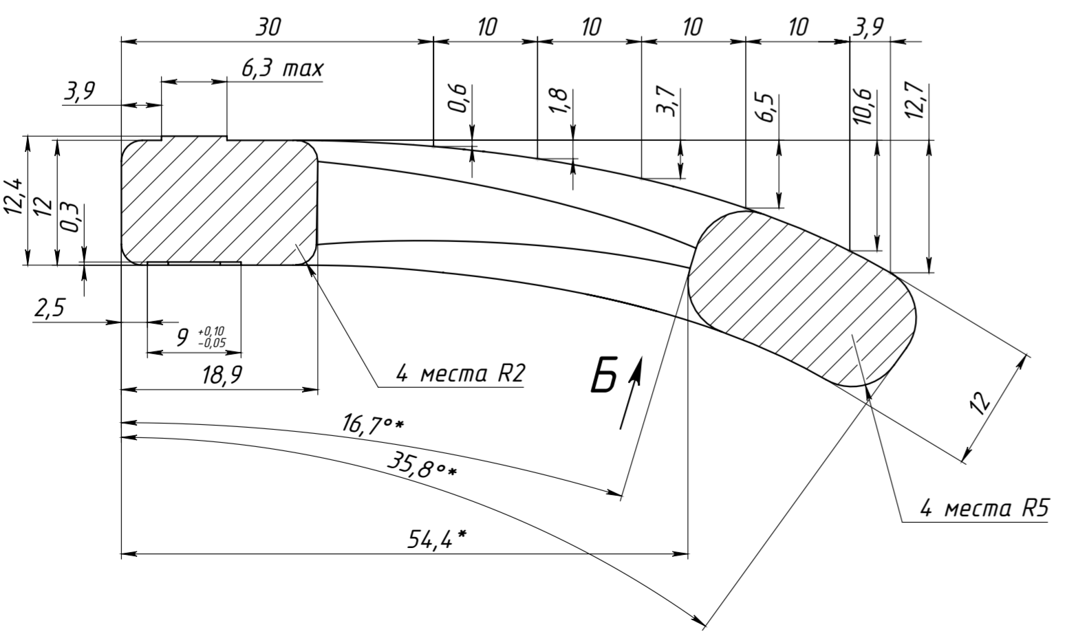
A-A (2 : 1)
