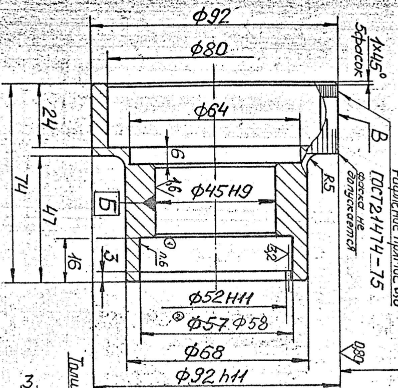
Разбертка поверхности В M 1:1
