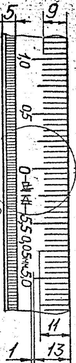
Разбертка поверхности В M 1:1
