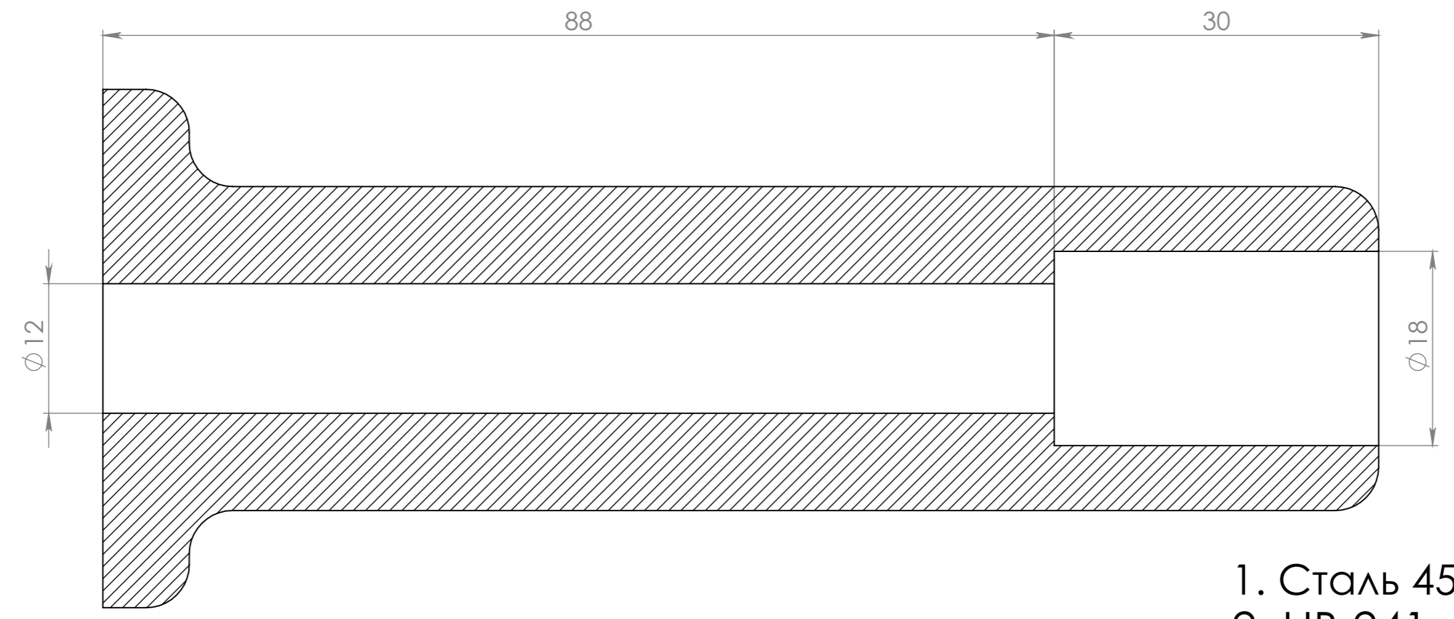
СЕЧЕНИЕ А-А МАСШТАБ 2 : 1
