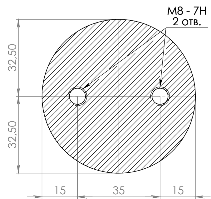
СЕЧЕНИЕ А-А МАСШТАБ 1 : 1
