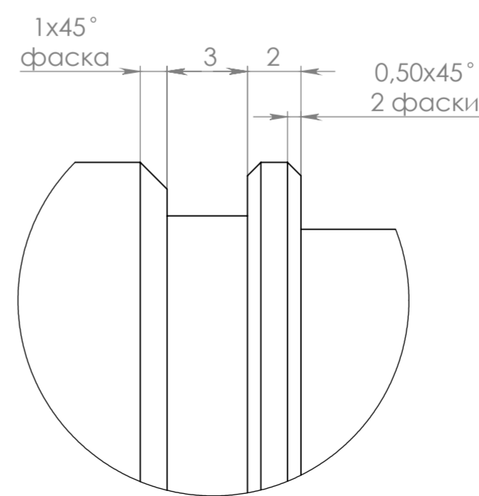
МЕСТНЫЙ Г МАСШТАБ 5 : 1
