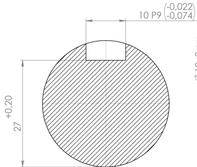
СЕЧЕНИЕ Б-Б МАСШТАБ 2 : 1
