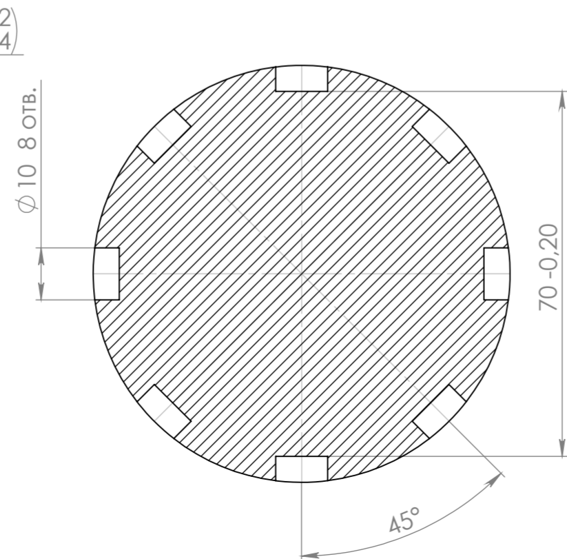
СЕЧЕНИЕ В-В МАСШТАБ 1 : 1
