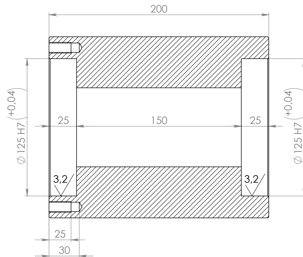
СЕЧЕНИЕ А-А МАСШТАБ 1 : 2
