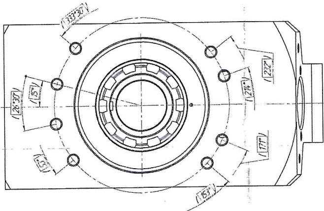
Рис. 3 (1:2,5) остальное см. УШЕМ 05.03.10.00.001
