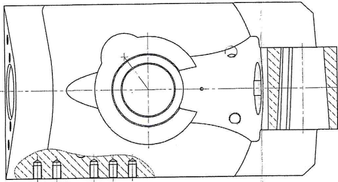
В (Рис. 4) (1:2,5) остальное см. УШЕМ 05.03.10.00.001
