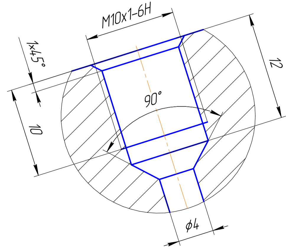
Б(4:1)
