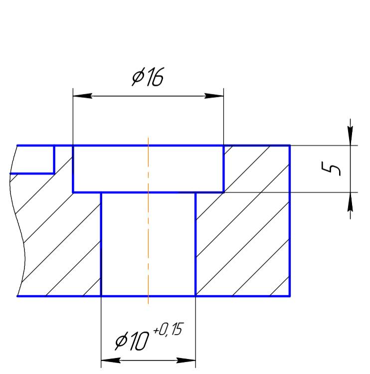
В-В(2,5:1)
