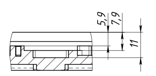
Р-Р (1:1)
