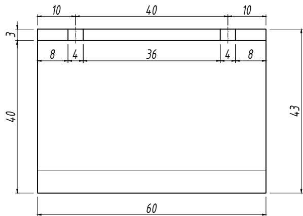
Разрез 2-2
