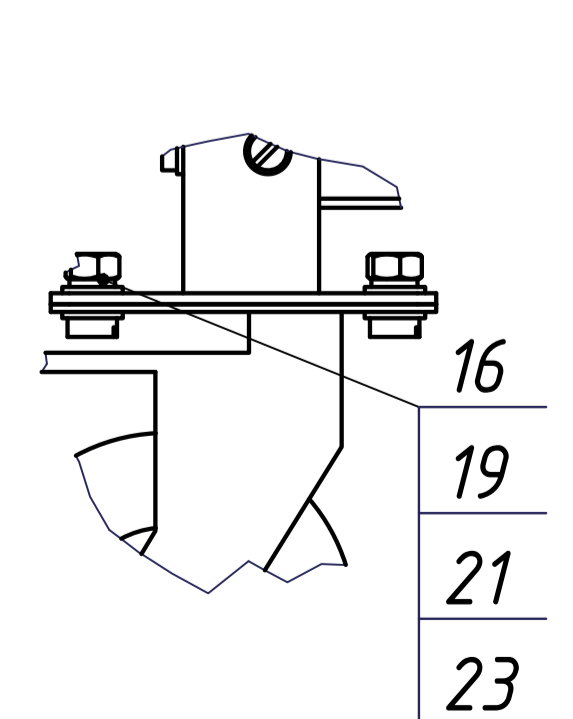
Б (1:2) 4 места
