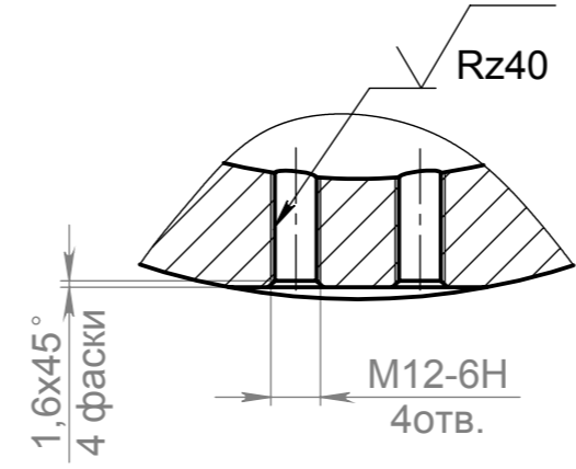
В-В (1 : 2)
