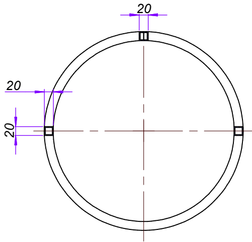
A-A ( 1 : 6 )
