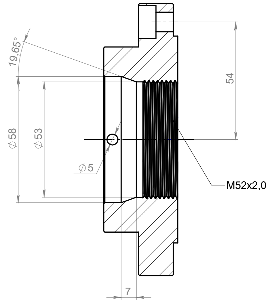
B-B (1 : 1)
