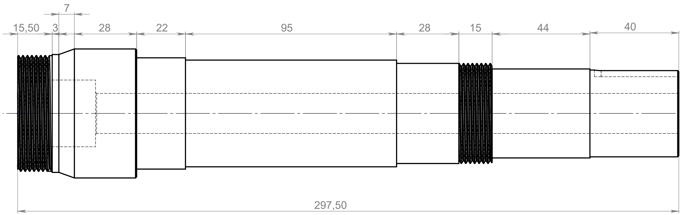
A-A (1 : 1)
