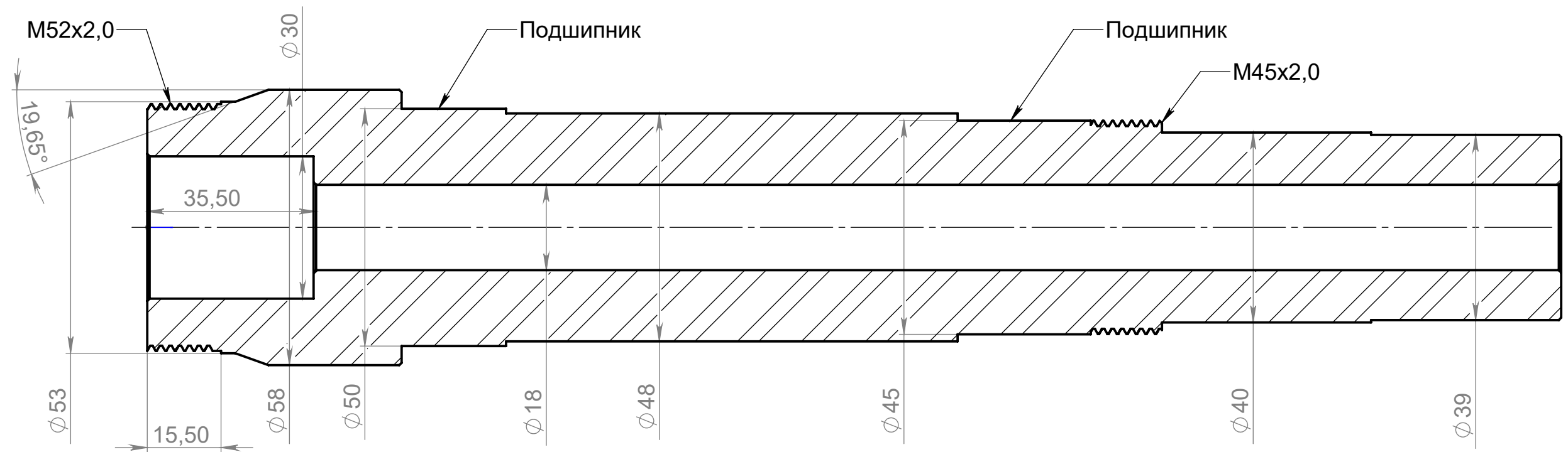
A-A (1 : 1)
